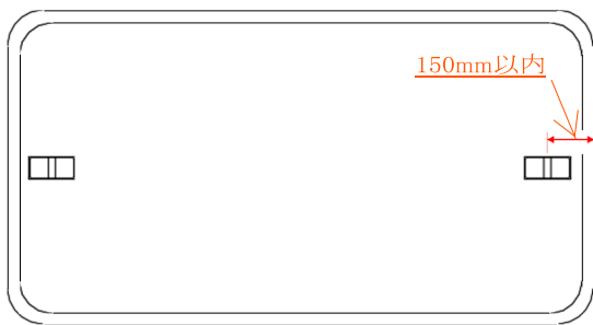
図1-2 角型鉄蓋(J型フック溝)
